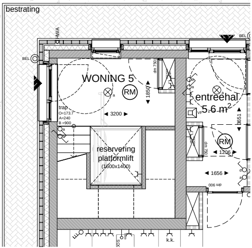
plattegrond begane grond 1:100
